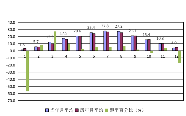
图 1 2018 年逐月平均气温值比较 (单位:℃)
