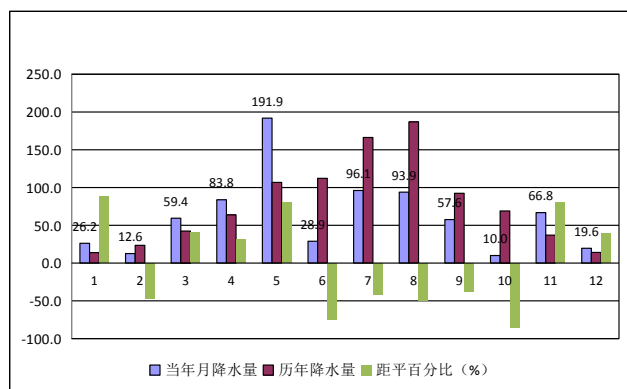
图 2 2018 年逐月降水量比较 (单位:mm)
