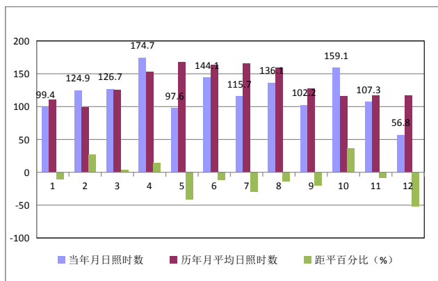
图3 2018年逐月日照时数距平分布(单位:h)
